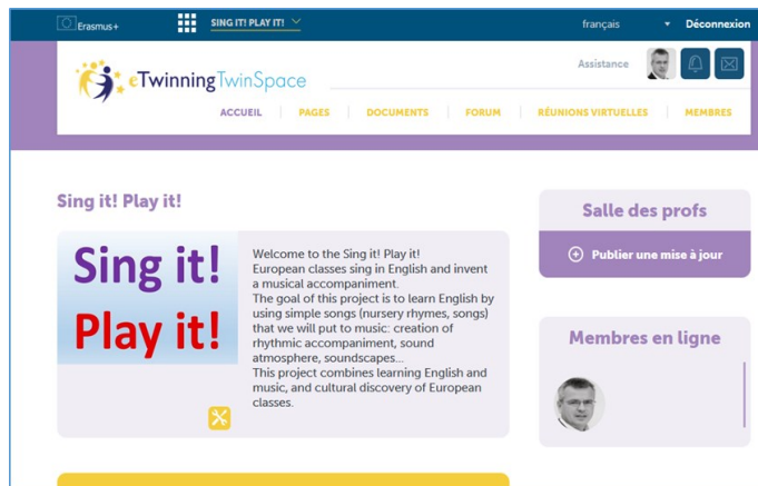
page d'accueil
